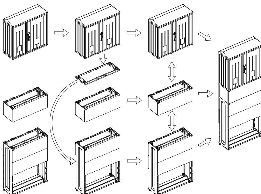
Obudowa OT + Kieszeń fundamentu FKO + Fundament OF OT enclosures + base for pedestal FKO + pedestal OT F Gehäuse OT + Kabelgehäuse FKO + Sockel OT F Корпус OT + Корпус фундамента FKO + Фундаментная подставка OT F
