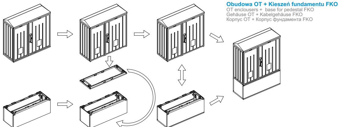
Obudowa OT + Fundament OT F OT enclosures + pedestal OT F Gehäuse OT + Sockel OT F Корпус OT + / Фундаментные подставки OT F
