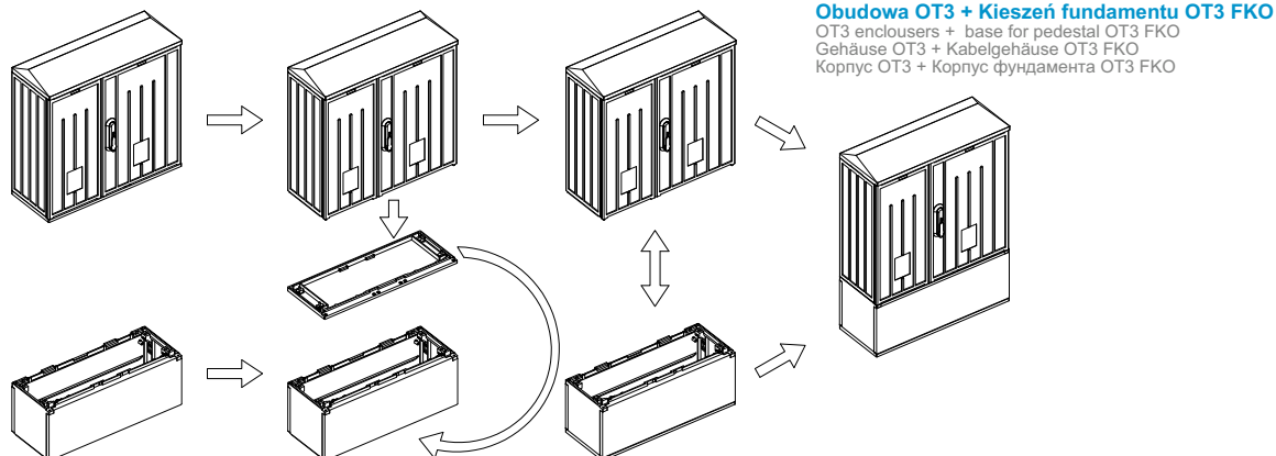
Obudowa OT3 + Fundament OT3 F OT3 enclosures + pedestal OT3 F Gehäuse OT3 + Sockel OT3 F Корпус OT3 + / Фундаментные подставки OT3 F
