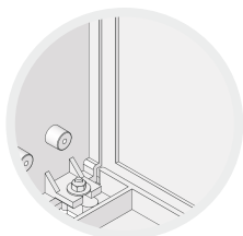
Typ B (brak izolatora na plecach) Type B (no insulator in the back wall) Typ B (kein Isolator auf der Rückseite) Тип В (отсутствие изолятора на задней стене корпуса)
