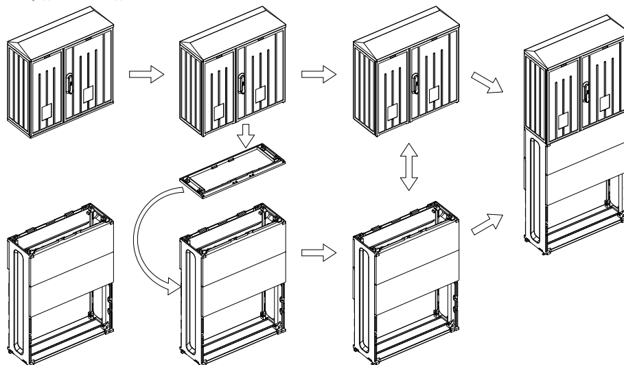
Obudowa OT3 + Kieszon fundamentu OT3 FKO + Fundament OT3 F OT3 enclosures + base for pedestal OT3 FKO + pedestal OT3 F Gehäuse OT3 + Kabelgehäuse OT3 FKO + Sockel OT3 F Корпус OT3 + Корпус фундамента OT3 FKO + Фундаментная подставка OT3 F
