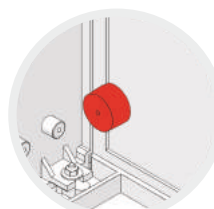
Izolator [F4] z otworem \varnothing 4 służący do montażu elementów za pomocą wkrętów
