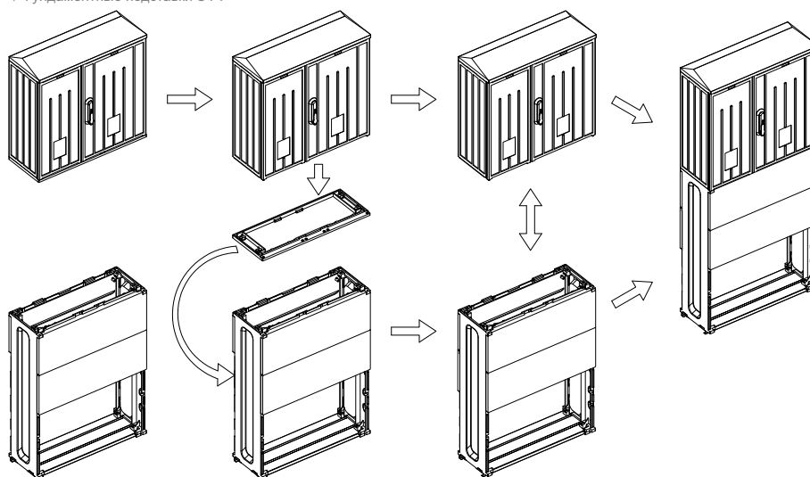
Obudowa OT + Kieszeń fundamentu FKO + Fundament OF OT enclosures + base for pedestal FKO + pedestal OT F Gehäuse OT + Kabelgehäuse FKO + Sockel OT F Корпус OT + Корпус фундамента FKO + Фундаментная подставка OT F
