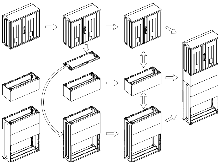
Obudowa OT3 + Kieszon fundamentu OT3 FKO + Fundament OT3 F OT3 enclosures + base for pedestal OT3 FKO + pedestal OT3 F Gehäuse OT3 + Kabelgehäuse OT3 FKO + Sockel OT3 F Корпус OT3 + Корпус фундамента OT3 FKO + Фундаментная подставка OT3 F
